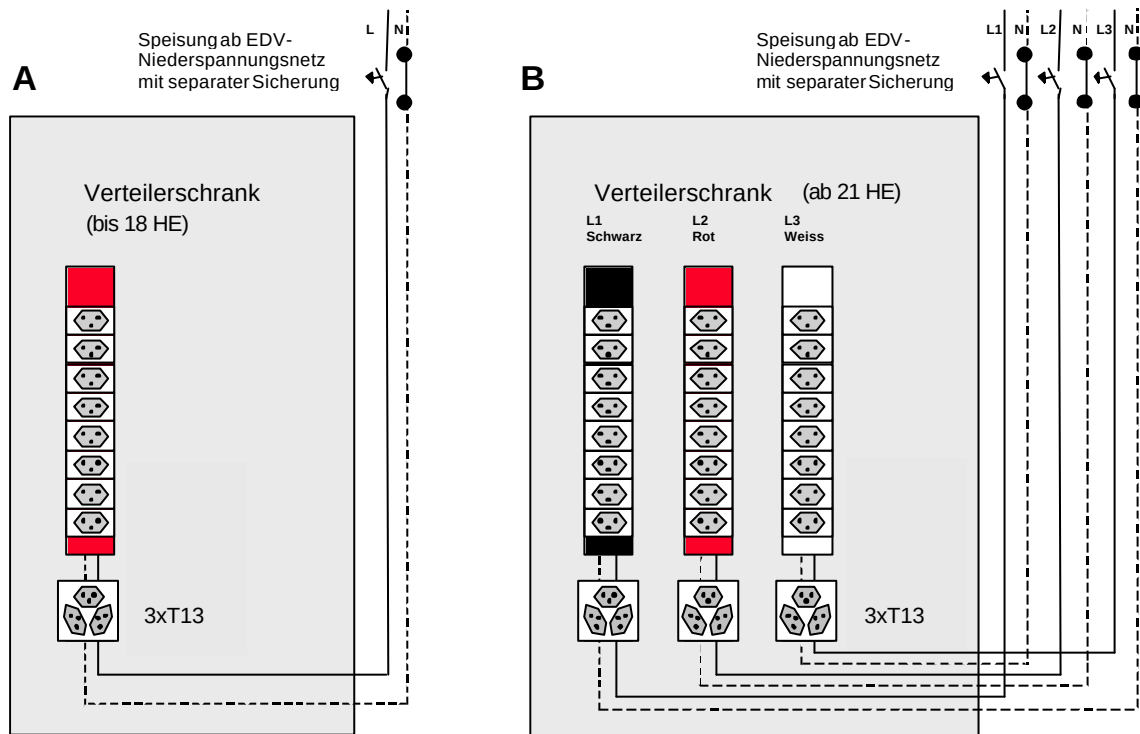
Abbildung 6: 230V-Anschluss eines Verteilers: A: eine getrennte Erschliessung B: drei getrennte Erschliessungen
