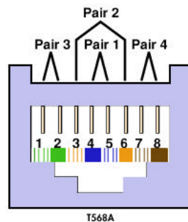
Abbildung 8: EIA/TIA-568-A-Standard
