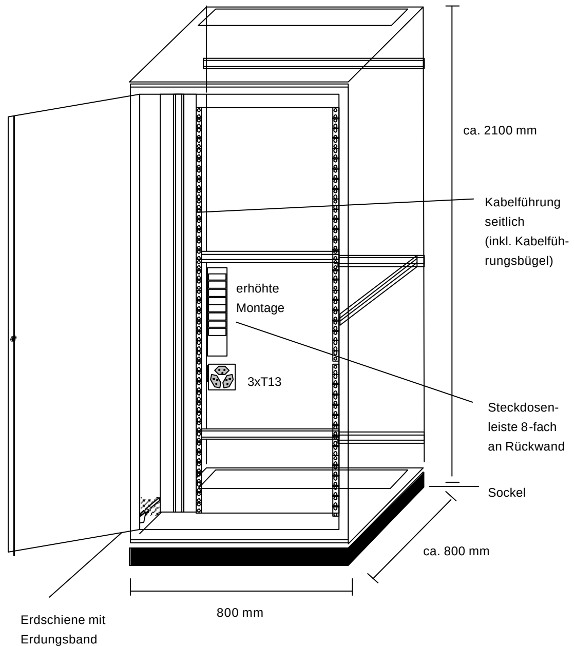
Abbildung 12: Prinzip 19"-Verteilerschrank
