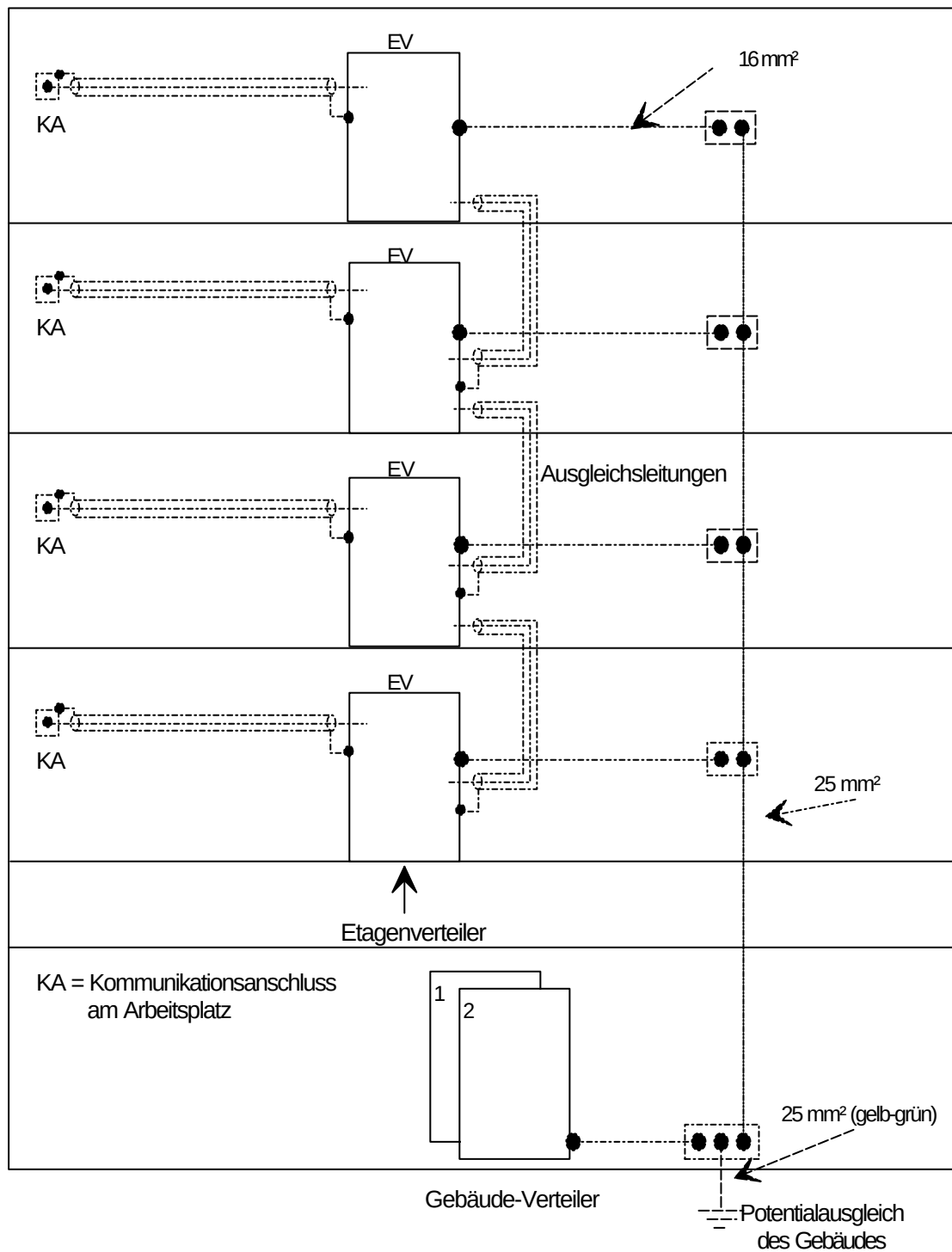
Abbildung 10: Kommunikationserde in einem Gebäude.
