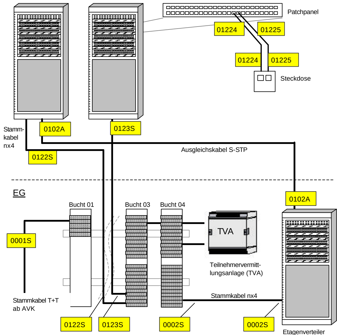
Abbildung 13: Kabelbeschriftungen
