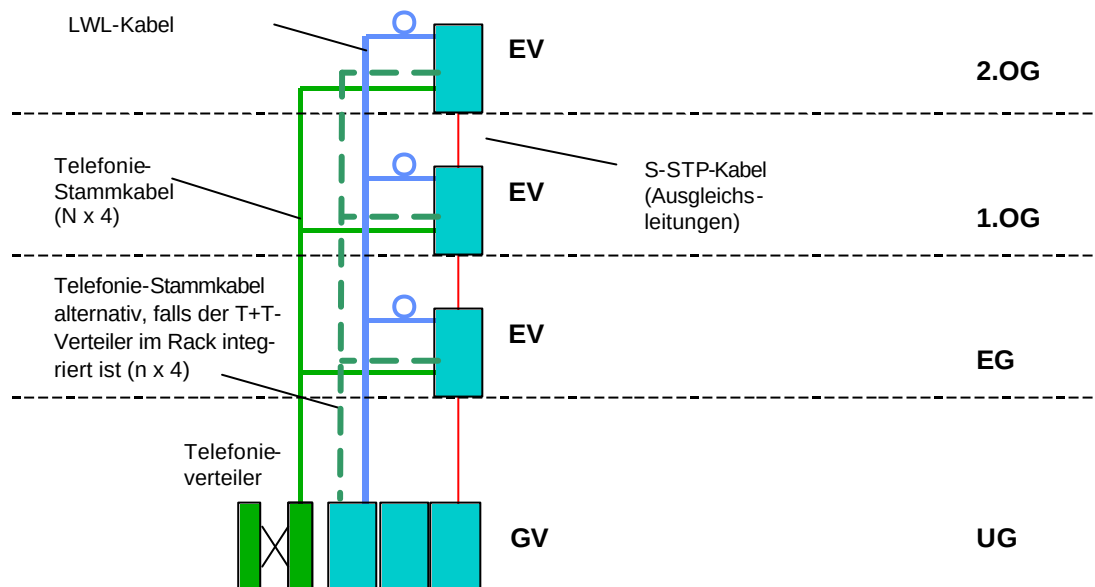
Abbildung 2: Struktur der Sekundärverkabelung.
