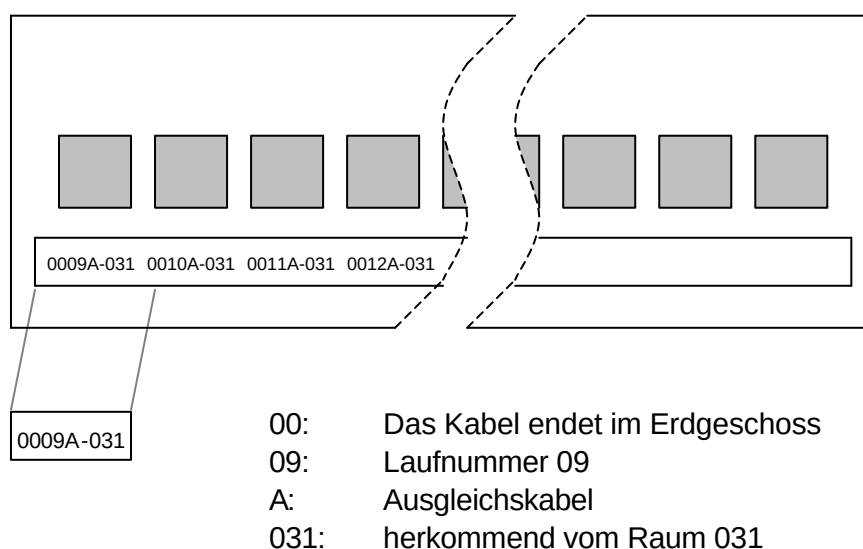
Abbildung 16: Beschriftung Verteilpanel-Dosen Ausgleichskabel
