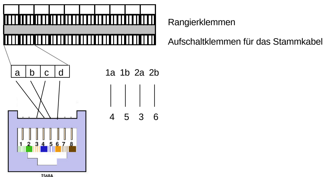
Abbildung 9: Verbindung VS83 zu RJ45
