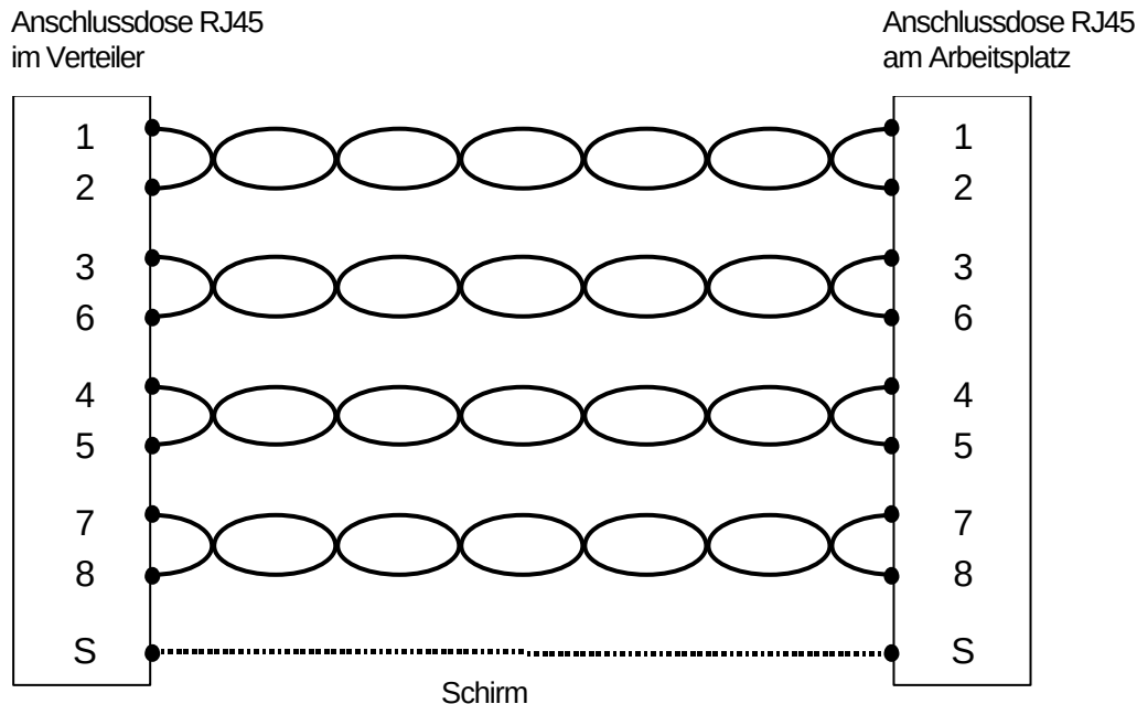
Abbildung 7: Anschlussschema RJ45.
