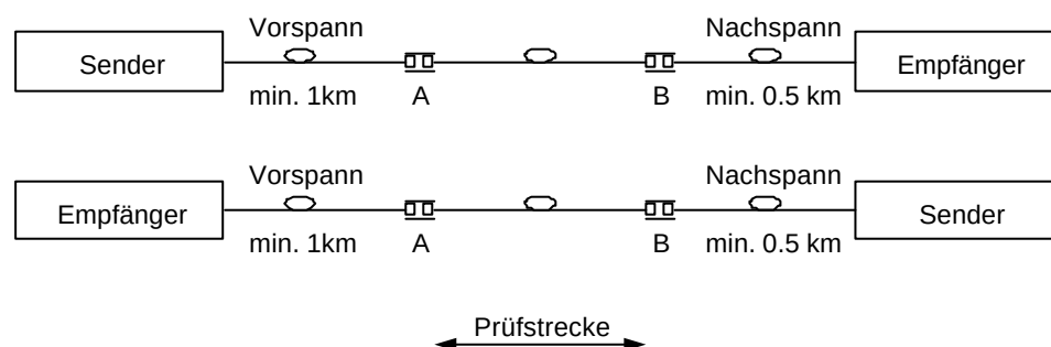
Abbildung 20: Leistungsmessung an einer LWL-Strecke.
