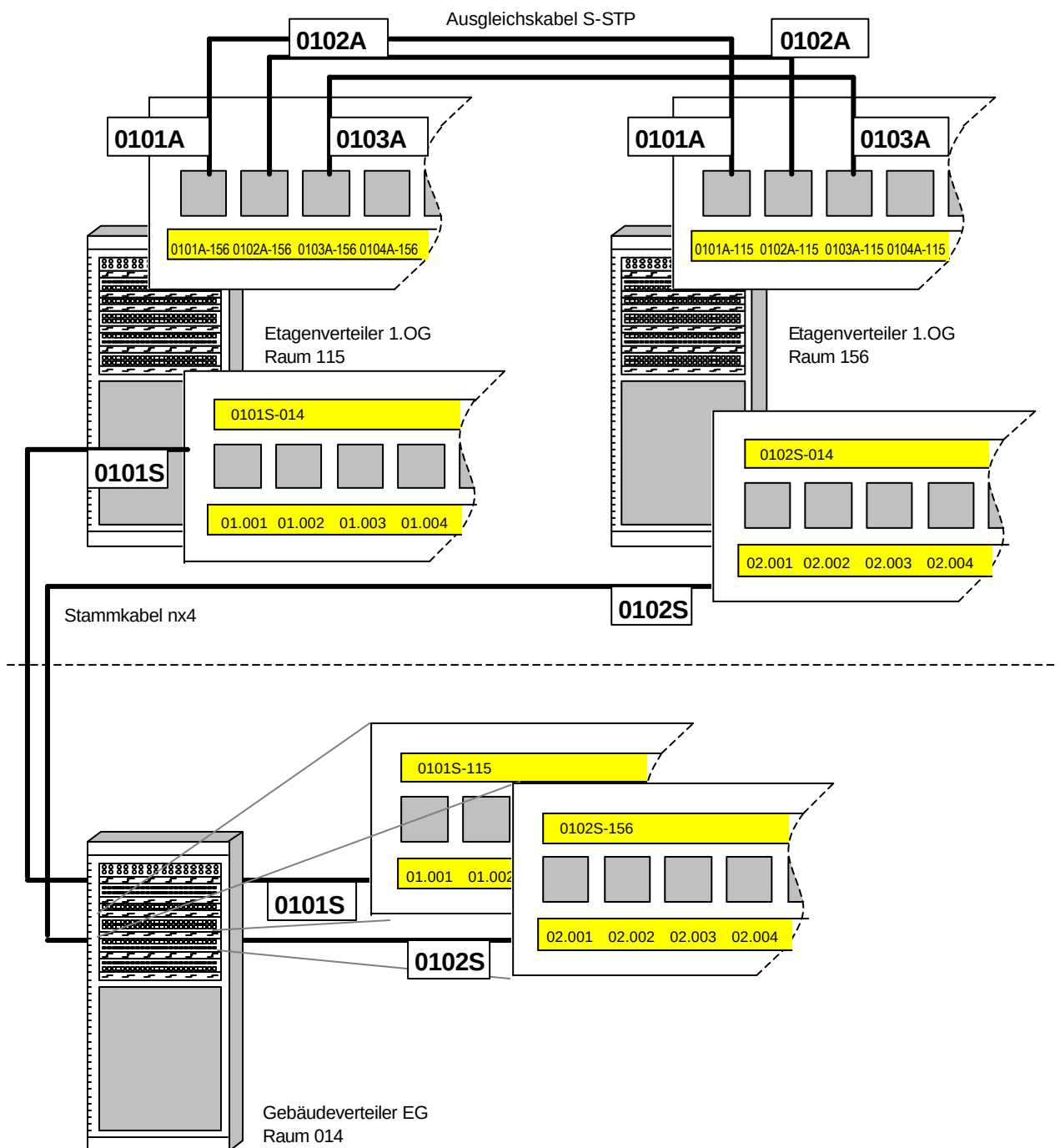
Abbildung 17: Beschriftung der Paneldosen im Sekundärsektor
