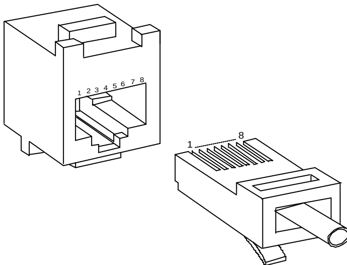
Abbildung 11: RJ45-Stecksystem.
