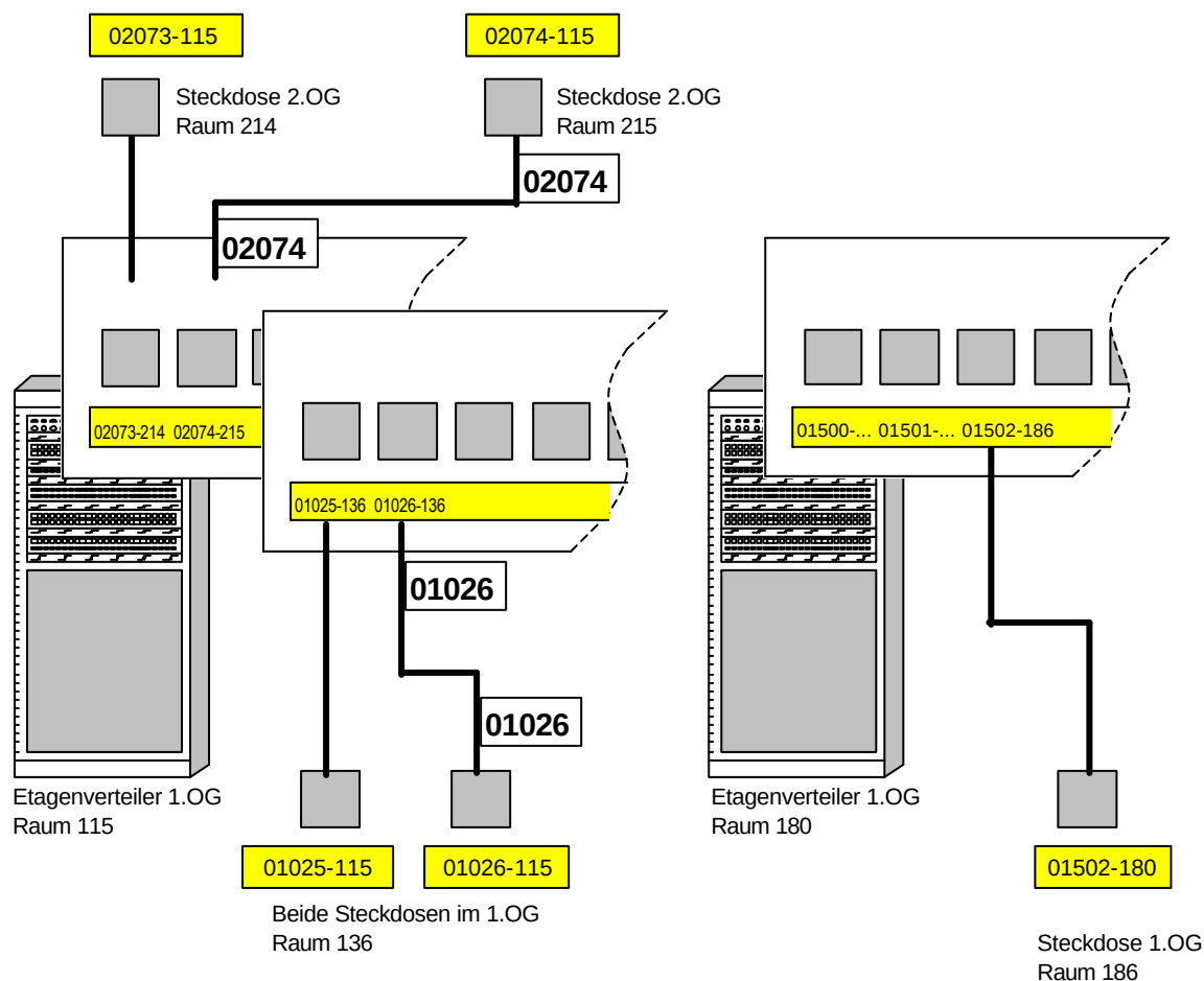
Abbildung 18: Beschriftung der Dosen im Tertiärsektor
