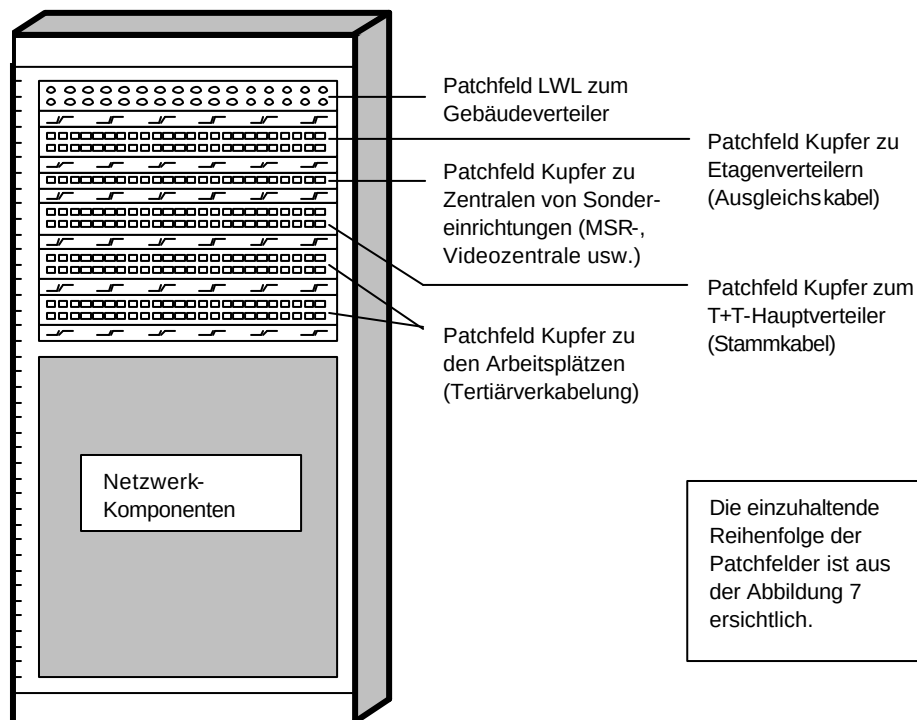
Abbildung 3: Verteiler-Layout.
